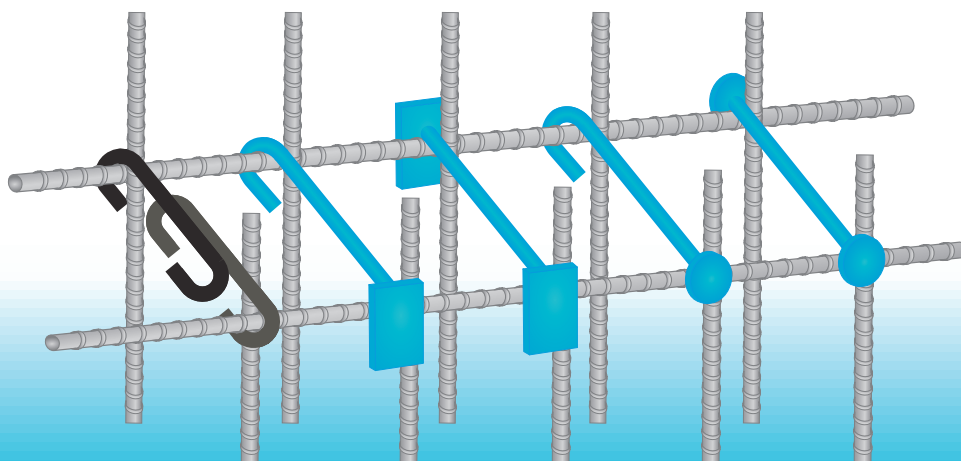
両端矩形プレート型 (I-Head-bar)
