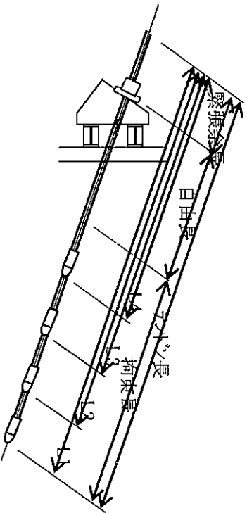
【寸法図】
